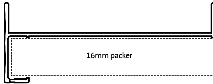
G03 - Return Jamb
