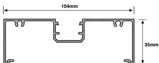
SIG 1008 - Main Frame
