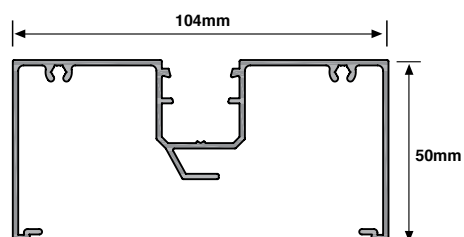
SIG 6008 - Main Frame
