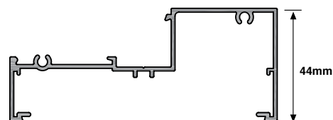
SIG 5002 - Sill / Transome
