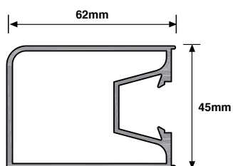
CD-311 - Narrow Hinge Stile
