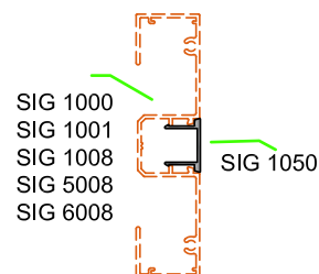
SIG 1050 - Pocket Filler
