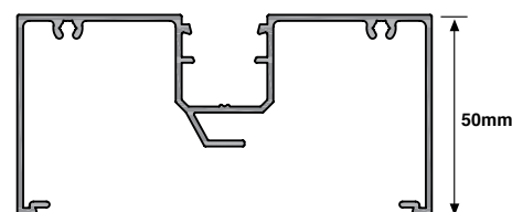
SIG 6008 - Door Frame 50mm
