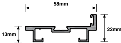
SIG 705 - 45mm Door Frame
