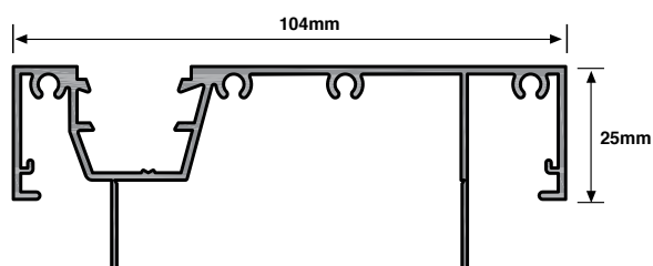
SIG 2001 - Main Frame
