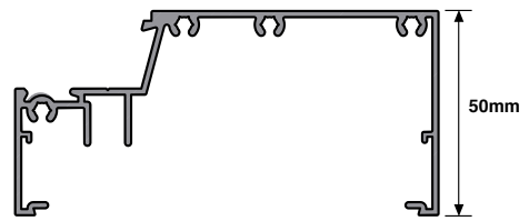
SIG 7002 - Sill / Transome
