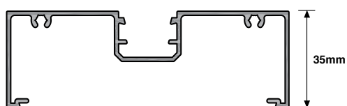
SIG 1008 - Door Frame 35mm
