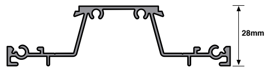
SIG 3002 - Sill / Transome
