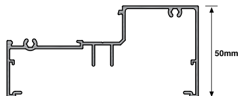
SIG 6002 - Sill / Transome
