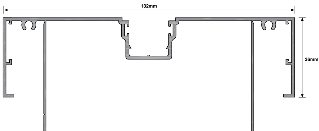
92mm Stud Framing
