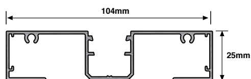
SIG 1000 - Main Frame
