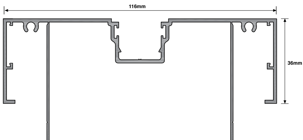
76mm Stud Framing
