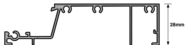
SIG 2002 - Sill / Transome
