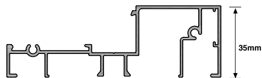
SIG 4002 - Sill / Transome
