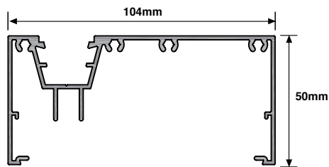
SIG 7001 - Main Frame
