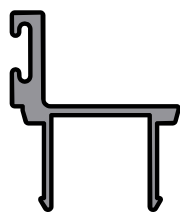
SIG 1035 - 35mm Door Stop
