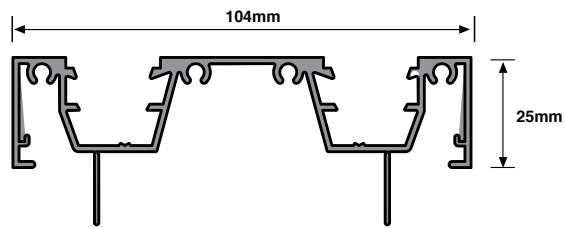
SIG 3001 - Main Frame
