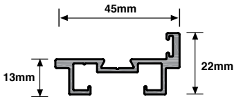
SIG 704 - 35mm Door Frame
