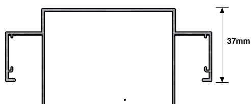
SIG 1006 - Shadowline Head
