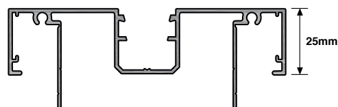
SIG 1001 - Main Frame
