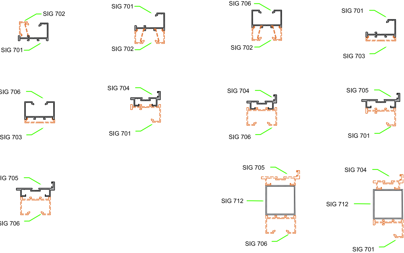
SIG 712 - 45mm Square Tube
