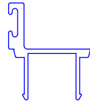
SIG 1035 35mm DOOR STOP
