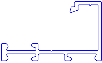
SIG 701 FRAME
