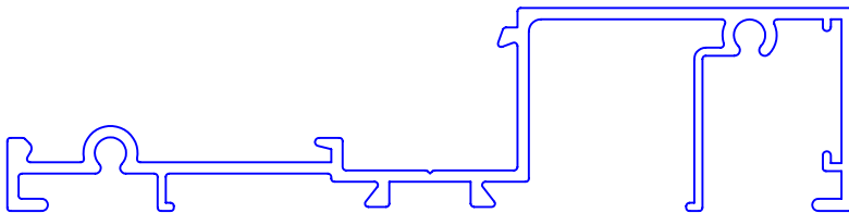
SIG 1002 SILL / TRANSOM
