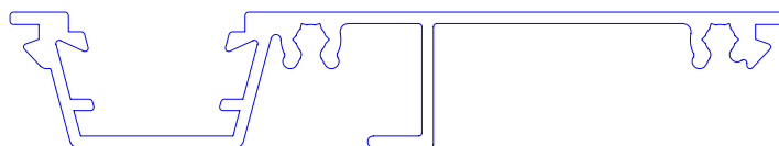
SIG 2009 GLAZING ADPTOR
