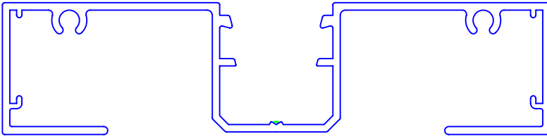
SIG 1000 MAIN FRAME
