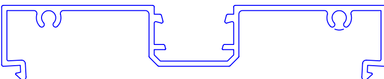
SIG 1004 TRANSOM
